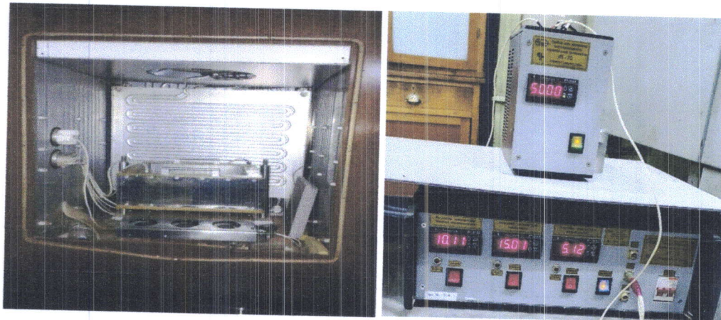
Рисунок 2 – Установа для визначення теплопровідності згідно з ДСТУ Б В.2.7-105-2000 (ГОСТ 7076-99)
