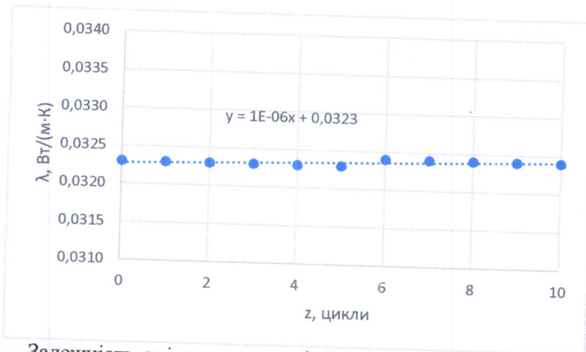
Рисунок 5 – Залежність зміни теплопровідності від циклічних впливів для зразків плит теплоізоляційних з екструдованого пінополістиролу (XPS) марки CARBON PROF виробництва ТОВ «ЗАВОД «СВІТОНДЕЙЛ»
