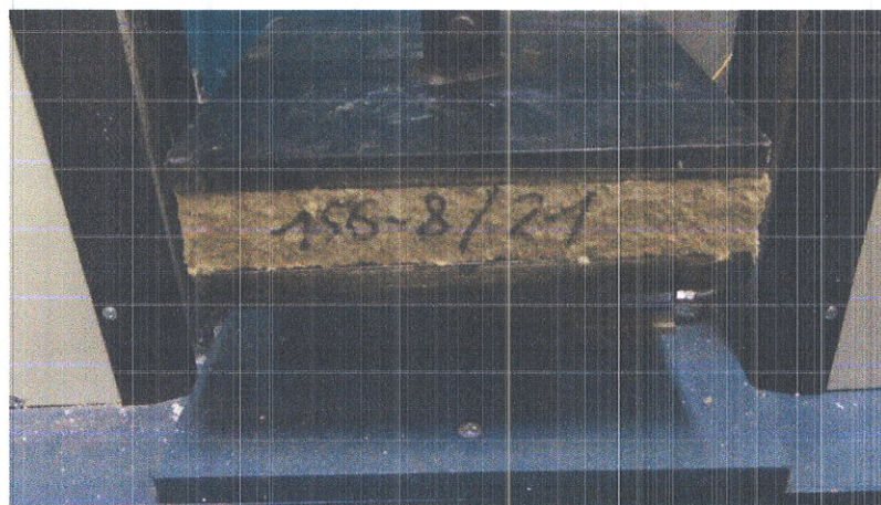
Рисунок 5 – Проведення випробування міцності на стиск при 10% деформації зразків теплоізоляційного матеріалу марки «THERMOWOOL ROOF N OPTIMA 110»
