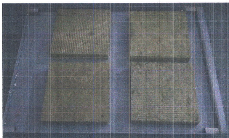
Рисунок 8 – Зволоження дослідних зразків теплоізоляційного матеріалу марки «THERMOWOOL ROOF V OPTIMA 180»
