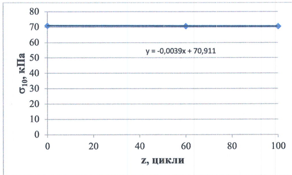
Рисунок 6 – Залежність міцності на стиск при 10% деформації від циклічних впливів зразків теплоізоляційного матеріалу марки «THERMOWOOL ROOF V OPTIMA 180»
