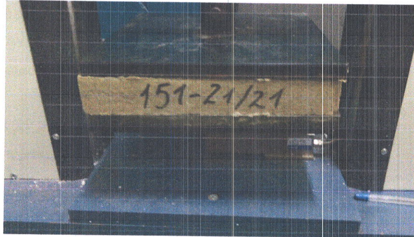
Рисунок 5 – Проведення випробування міцності на стиск при 10% деформації зразків теплоізоляційного матеріалу марки «THERMOWOOL ROOF V OPTIMA 180»
